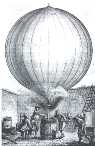
Denne tegning fra 1700-tallet viser fremstilling af brint (hydrogen) af jernspåner og svovlsyre.
